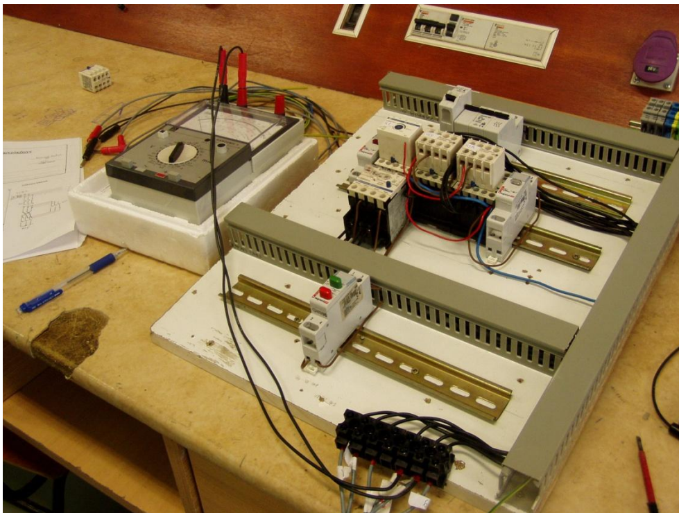
Kész munkadarab villamos bemérése
