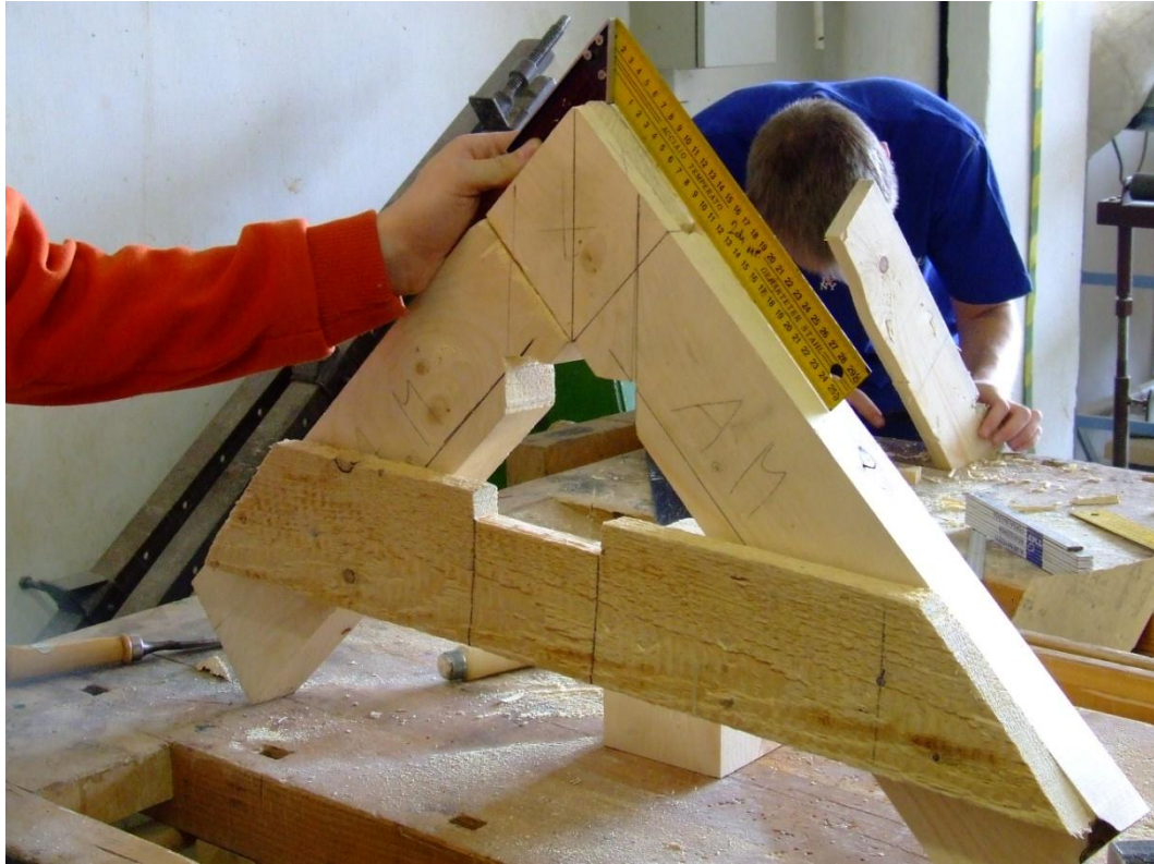
Tetőszerkezeti csomópont készítése
